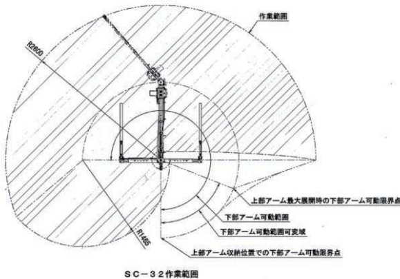
作業範囲(半径2,600mm)
