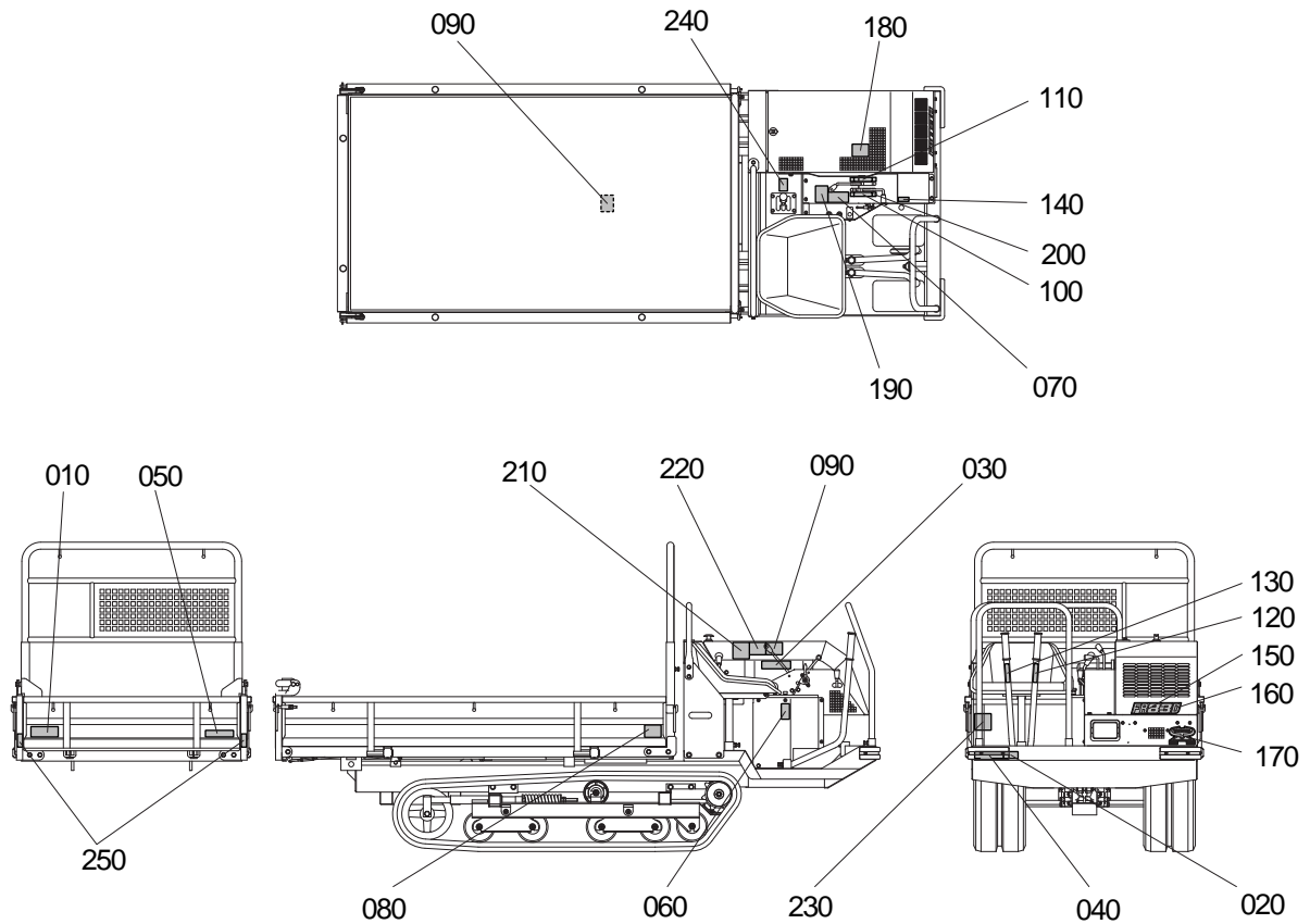
Fig.10 ラベル関係
