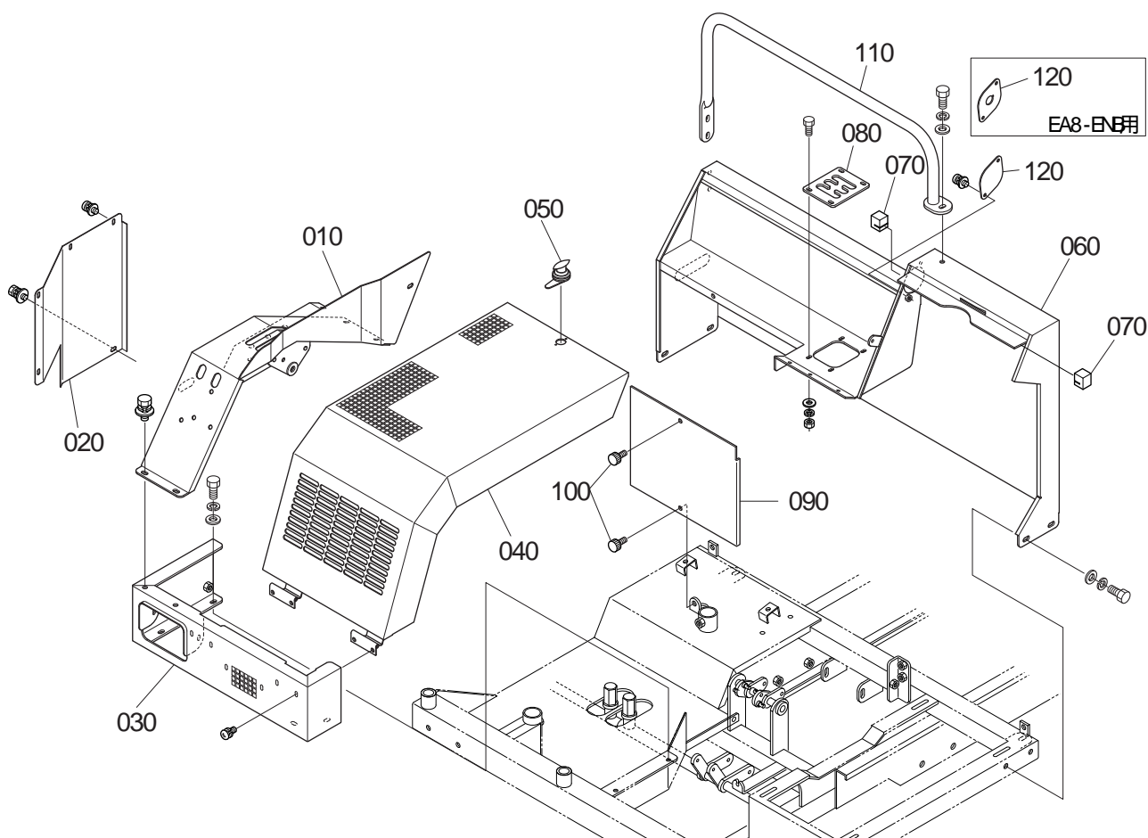
Fig.2 カバー関係
