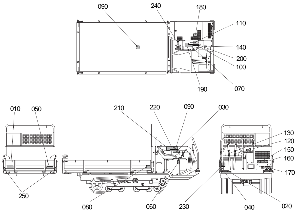
Fig.10 ラベル関係
