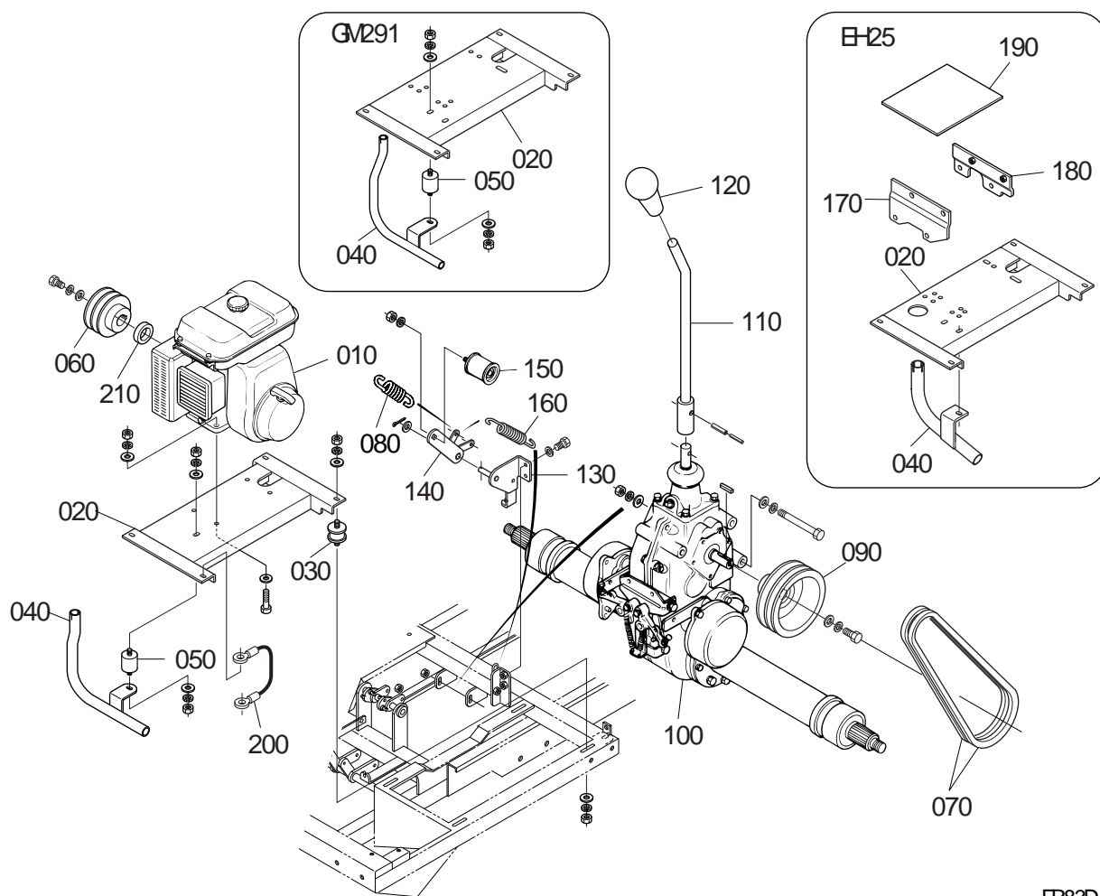
Fig.3 エンジン関係 -2
