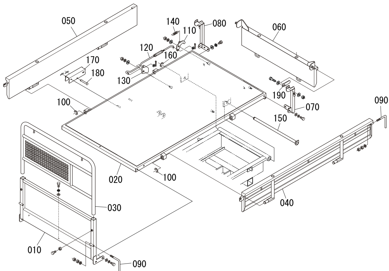
Fig. 9 荷箱関係
