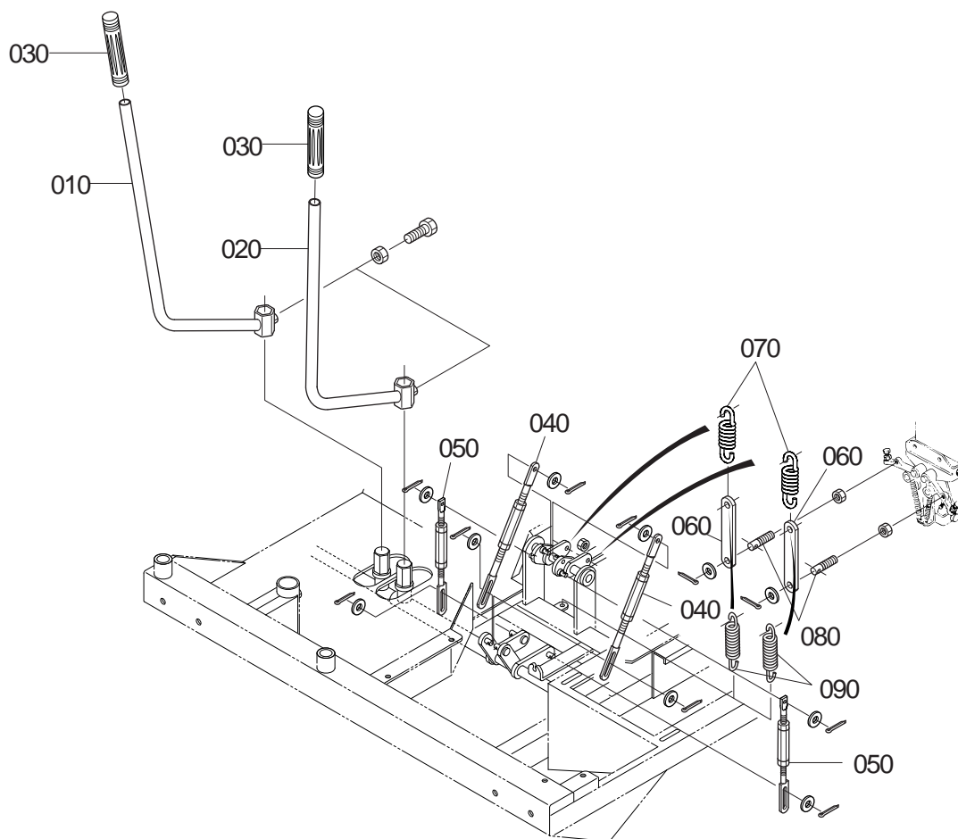
Fig.4 走行レバー関係
