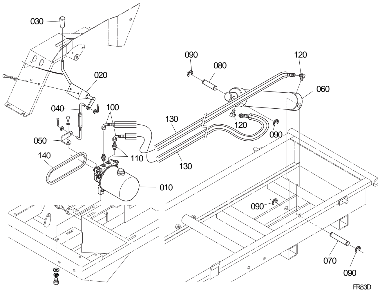
Fig.8 油圧関係
